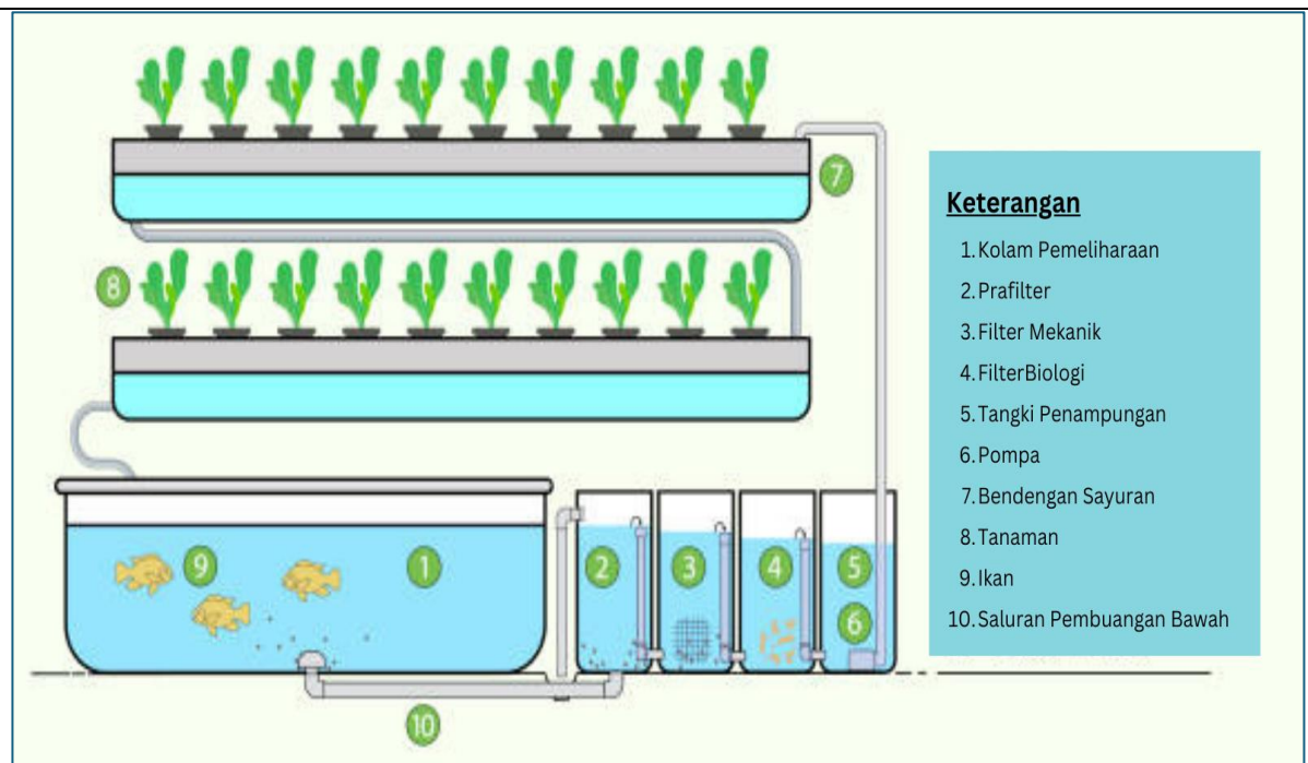
Gambar 2. Instalasi Aquaponik
